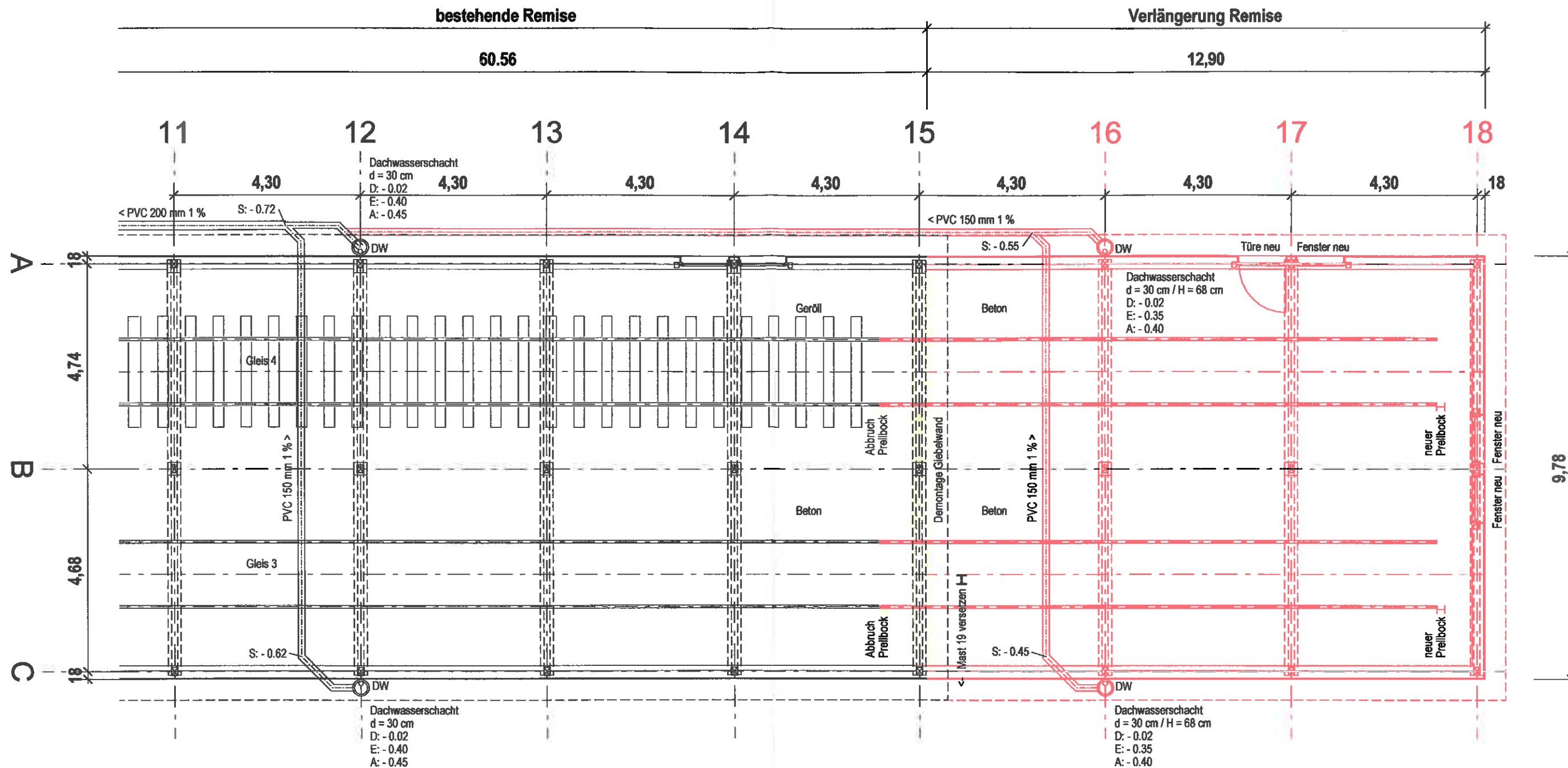
Grundriss Gebäude 2038
